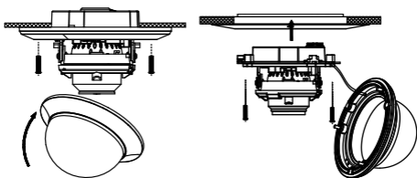
Рисунок 2-12 Установка камеры (Слева) Камера II типа (Справа) Камера III типа
